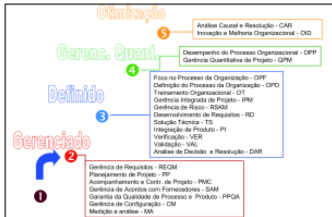
Figura 3 - Áreas de Processo por nível de maturidade CMMI em desenvolvimento de software
